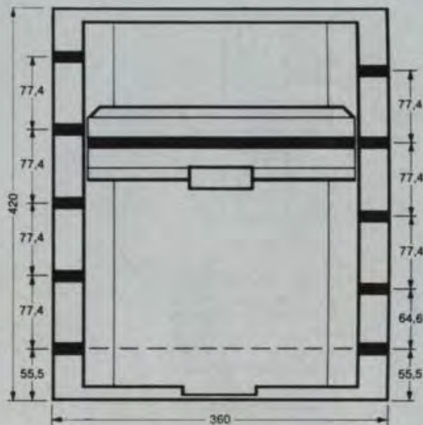
7294 Ferngesteuerte Schiebebühne
