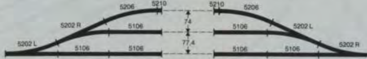
Gleisplan-Zeichenschablone 0209
